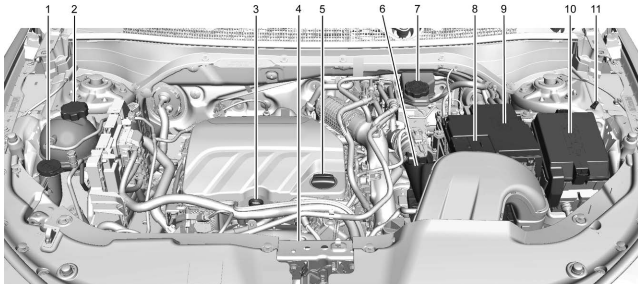
Motor 1.2L I3 (LBP)
